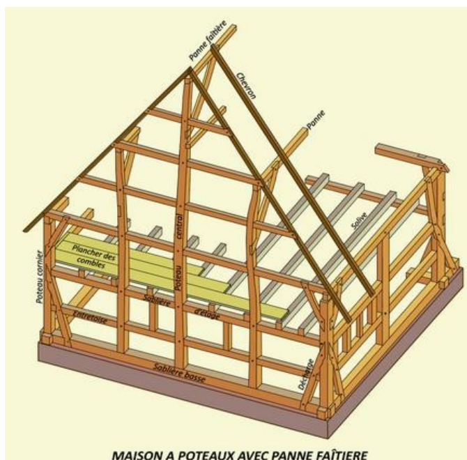
MAISON A POTEAUX AVEC PANNE FAÎTIÈRE
